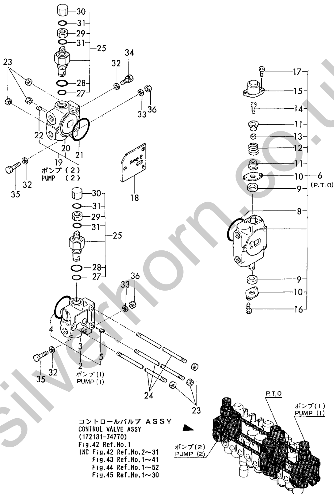
Fig. 42 コントロールバルブ(Pポート & P.T.O)(BIO) CONTROL VALVE (P PORT & P.T.O)
