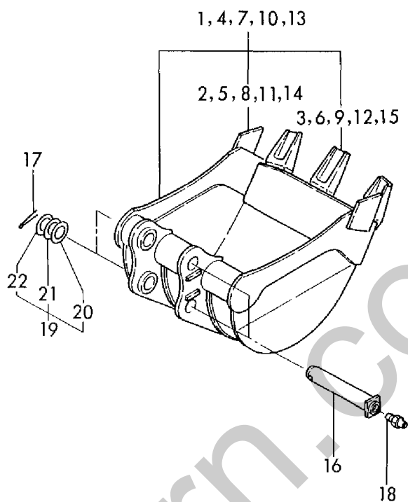
Fig. 58 バケット BUCKET
