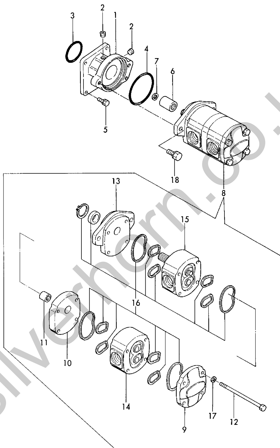
Fig. 31 ポンプ & ポンプマウント HYD. OIL PUMP & PUMP MOUNT
