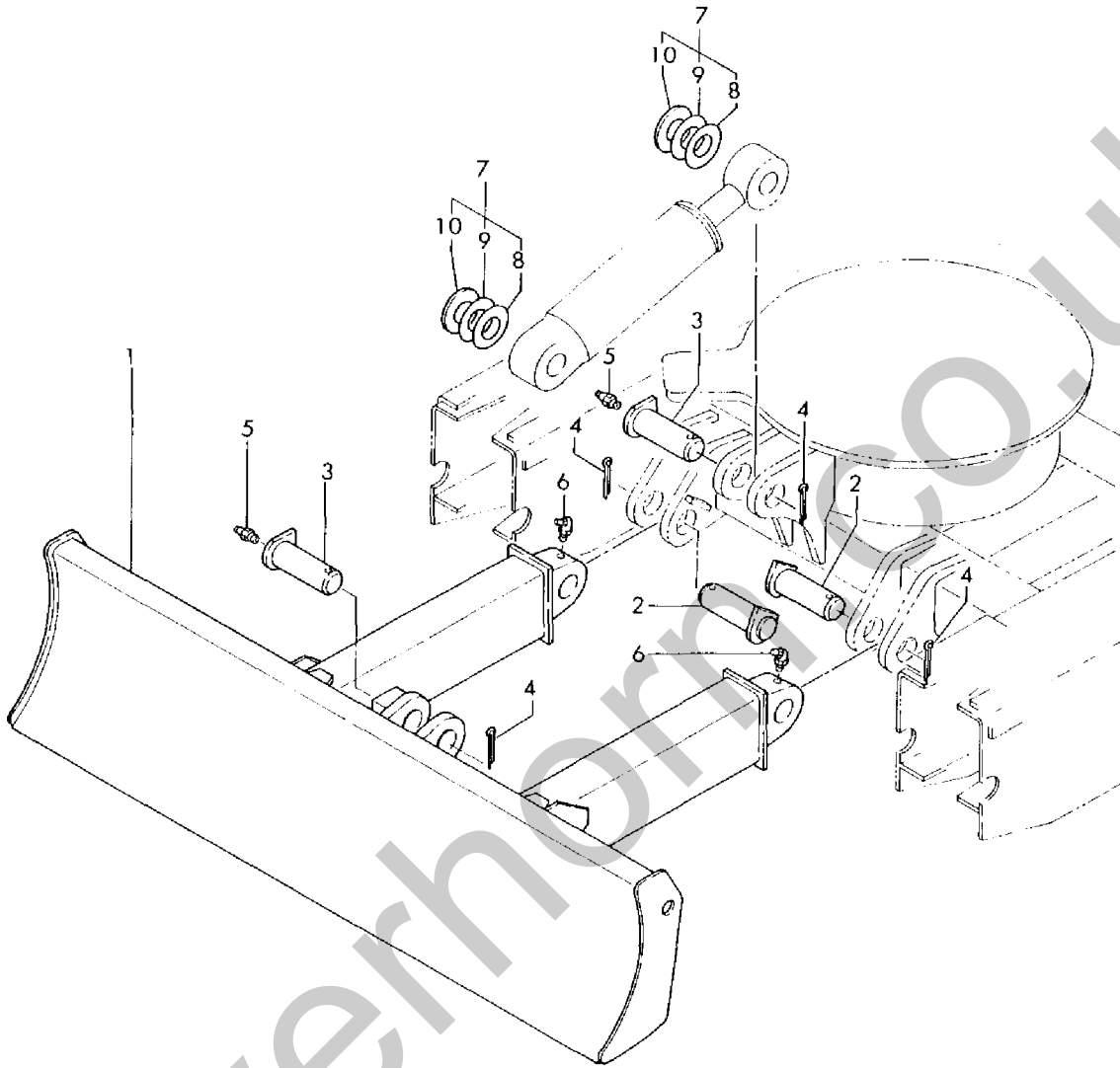
Fig. 57 ブレード BLADE
