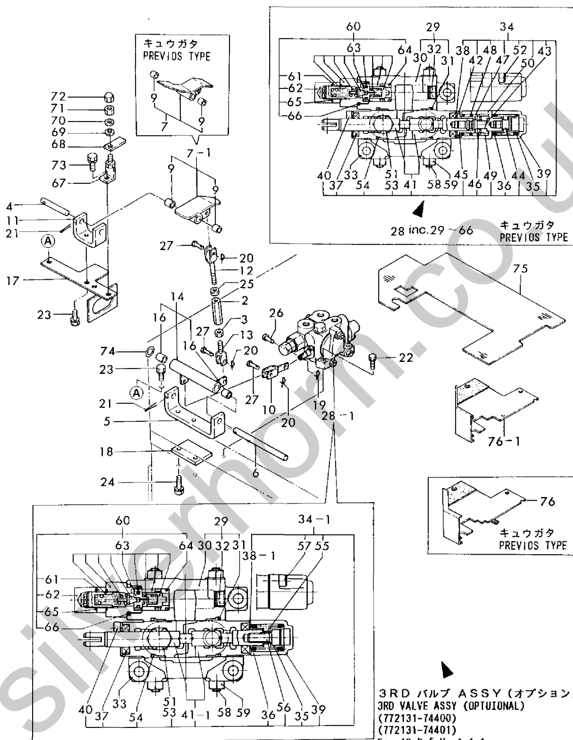
Fig. 46 サードバルブ コントロール (YB101) 3RD VALVE CONTROL
