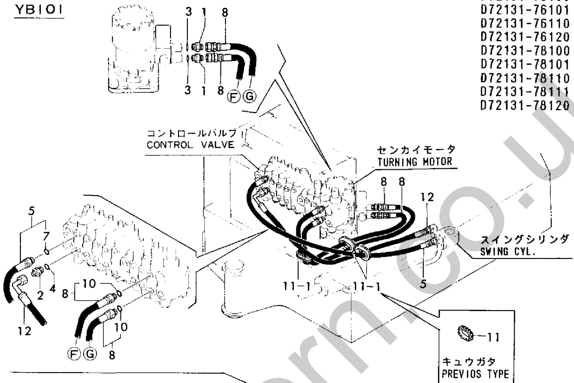
Fig. 49 ユアツハイカン(バルブモータ, スイング, P.T.O) HYD. OIL PIPING (VALVE-MOTOR, SWING, P.T.O)
