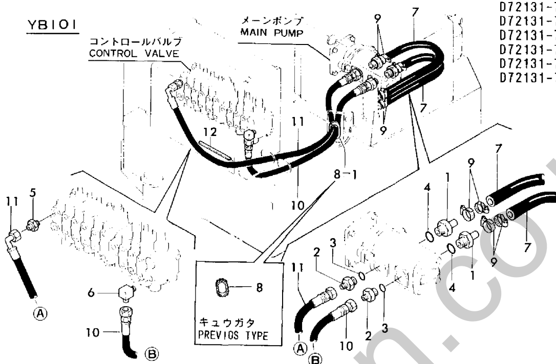
Fig. 48 ユアツハイカン (タンクーポンプバルブ) HYD. OIL PIPING (TANK-PUMP-VALVE)
