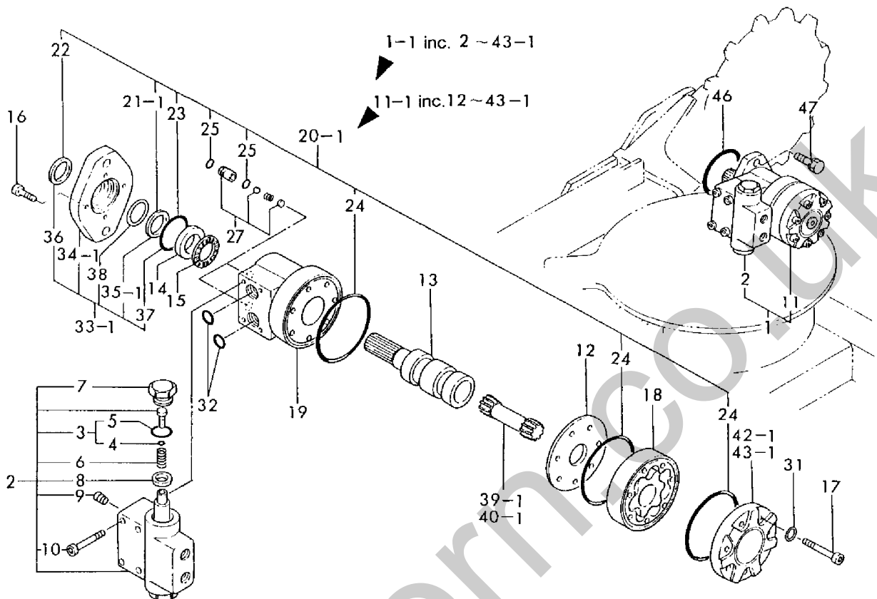
Fig. 38 ソウコウモータ DRIVING MOTOR
