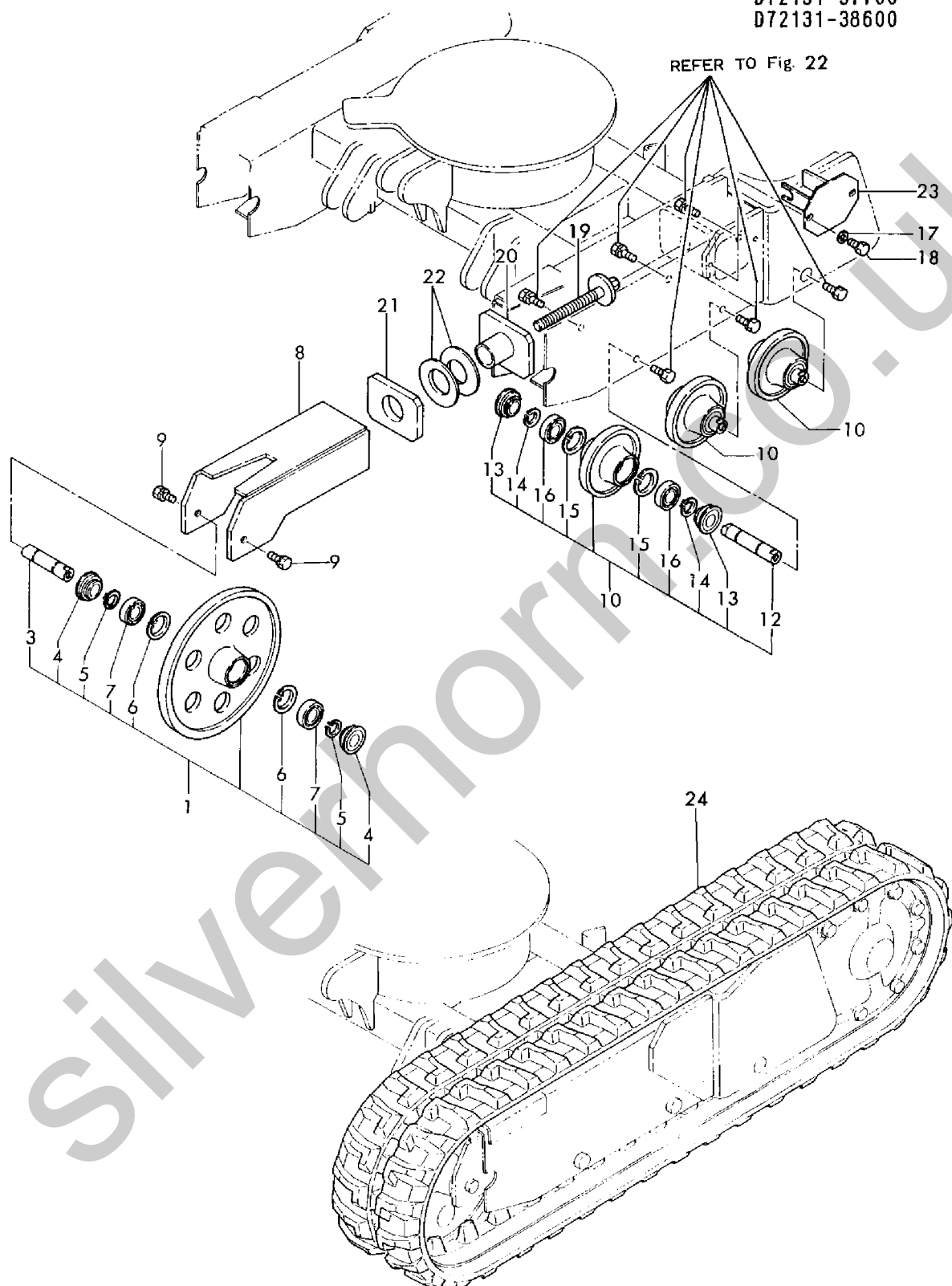
Fig. 14 アイドラ,トラックローラ & クローラ IDLER, TRACK ROLLER & CRAWLER
