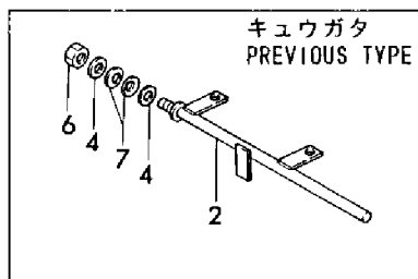
Fig. 21 サギョウレバーストップパ OPERATION LEVER STOPPER
