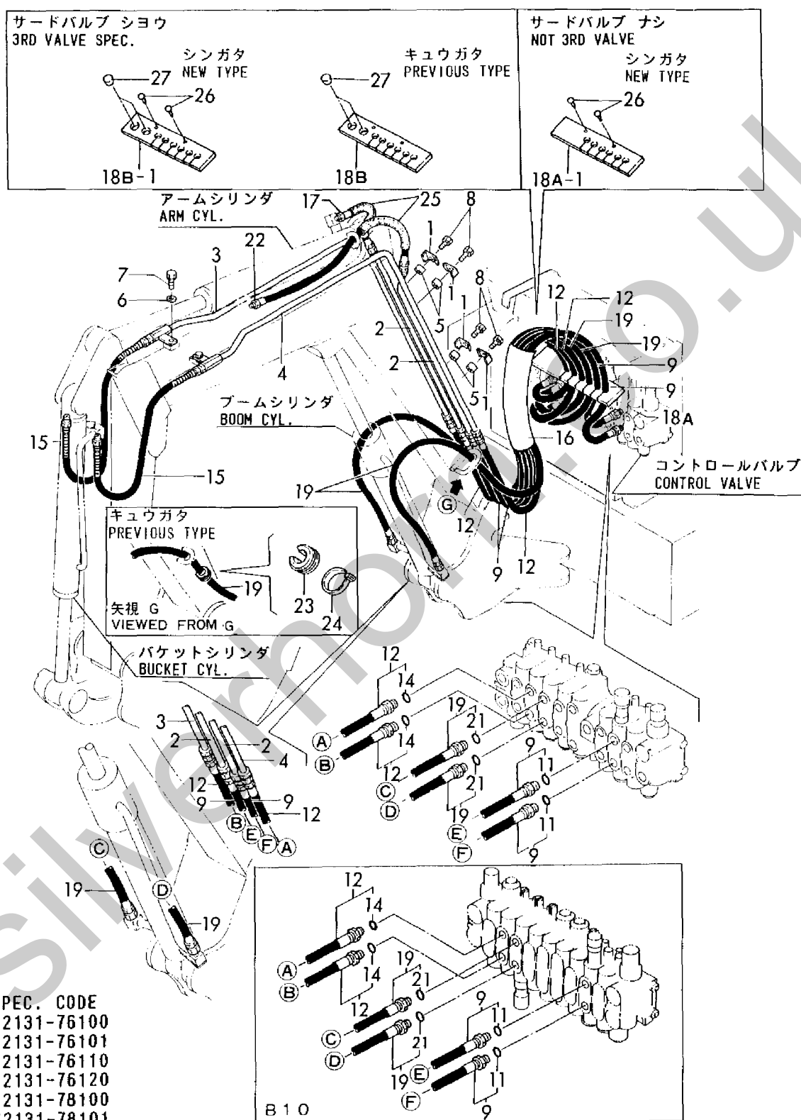
Fig. 53 ユアツハイカン(ブーム) HYD. OIL PIPING (BOOM)
