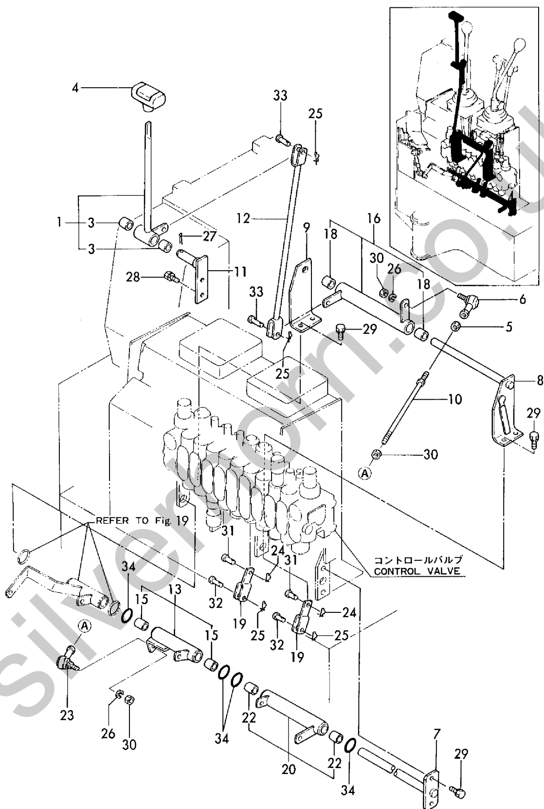
Fig. 15 ソウジュウソウチ(ブレード) (BIO) CONTROL EQUIPMENT (BLADE)
