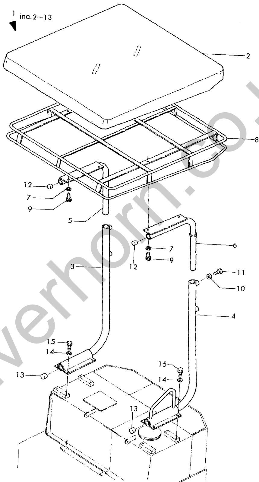
Fig. 30 キャンピ CANOPY
