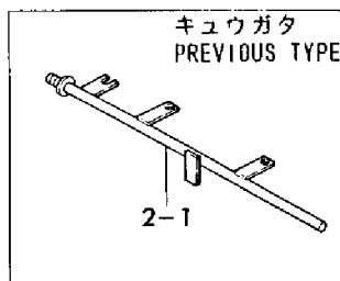
Fig. 21 サギョウレバーストップパ OPERATION LEVER STOPPER
