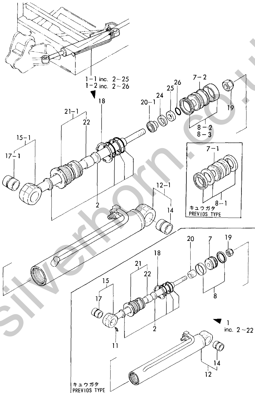
Fig. 37 スイング シリンダ SWING CYLINDER
