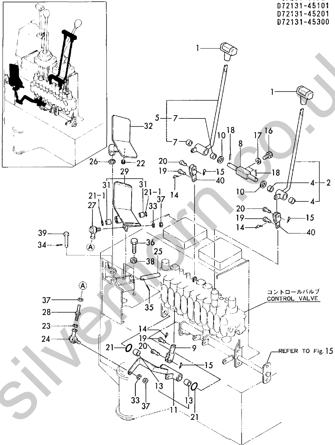
Fig. 19 ソウジュウソウチ(ソウコウ & スイング)(BIO) CONTROL EQUIPMENT (DRIVE & SWING)
