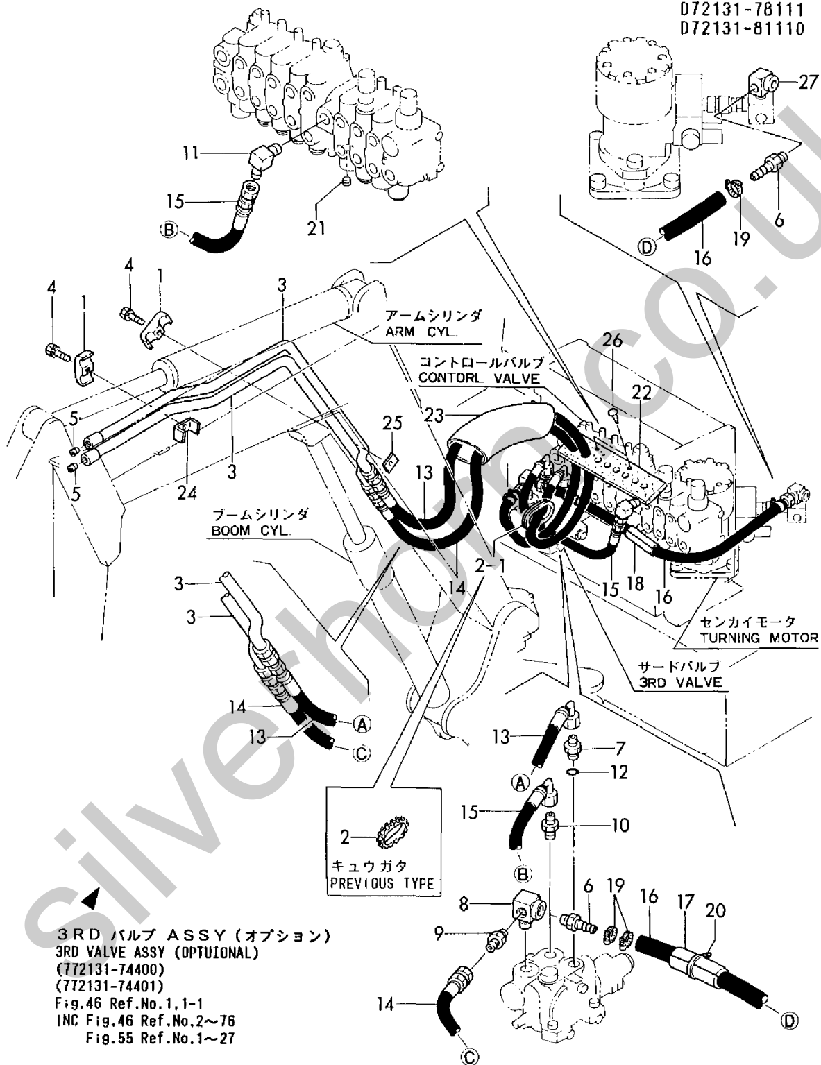
Fig. 55 サードバルブ ハイカン (YB101) 3RD VALVE OIL PIPING
