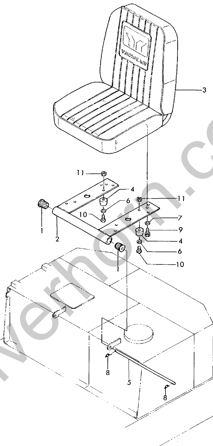
Fig. 27 シート (A) & シートマウント SEAT (A) & SEAT MOUNT
