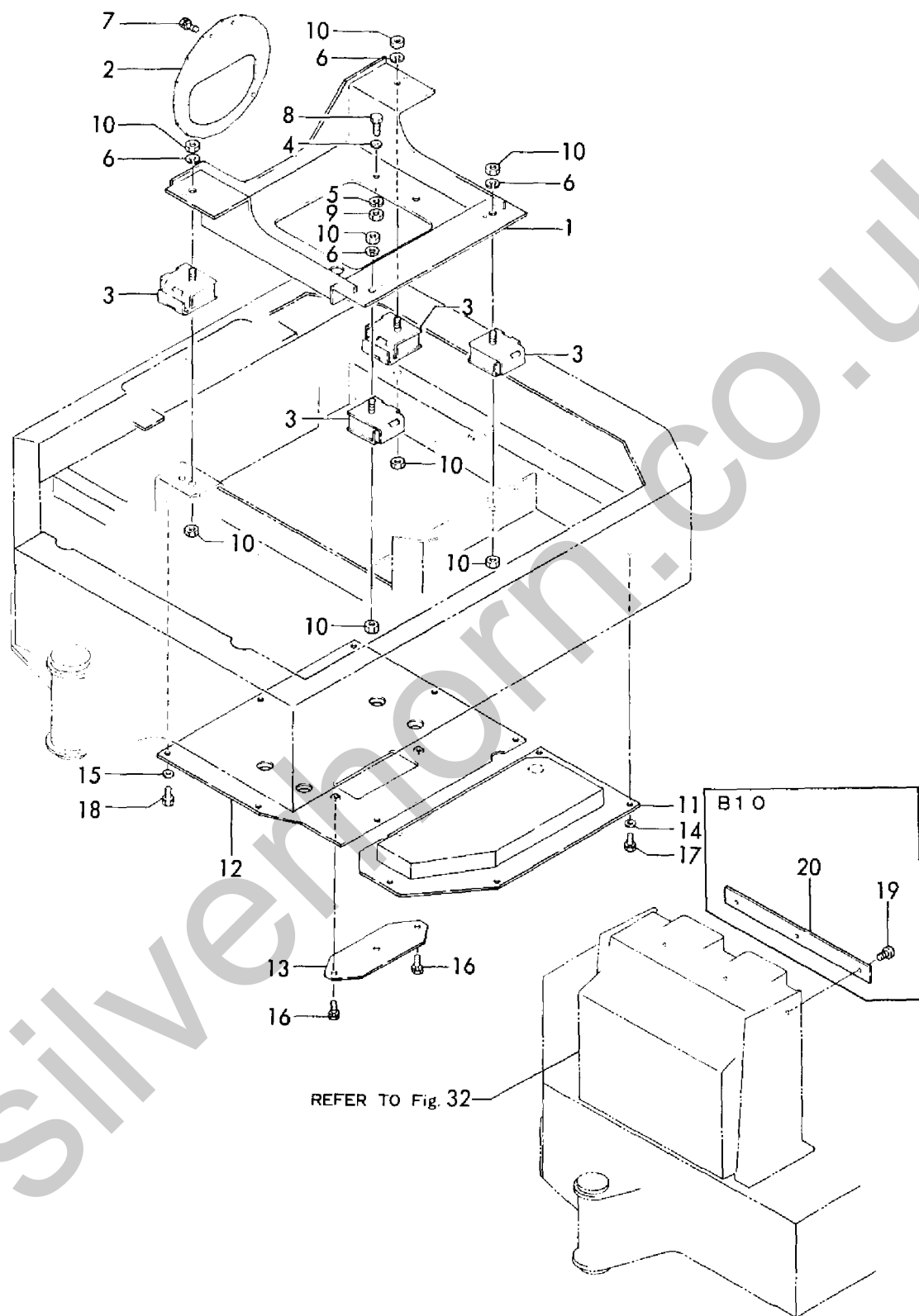
Fig. 8 エンジン マウント & カバー ENGINE MOUNT & COVER
